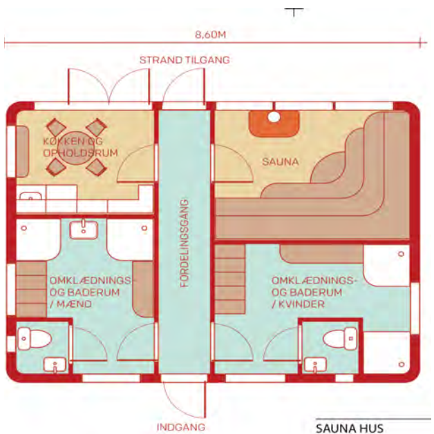
SAUNA HUS STUEPLAN 23-05-2021
